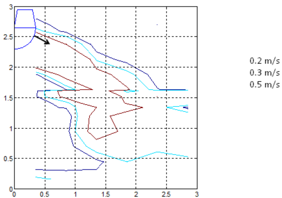
Kuva 3. Tasaopeuskäyrät yllämpöisellä tuloilmalla ( dt=+3^{\circ}\text{C} ). Ilmavirta 300 l/s. Vaaka- ja pystyakselien mitat metreinä.
